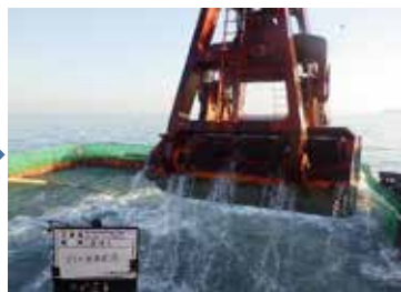
土運船運搬、揚土船接舷
